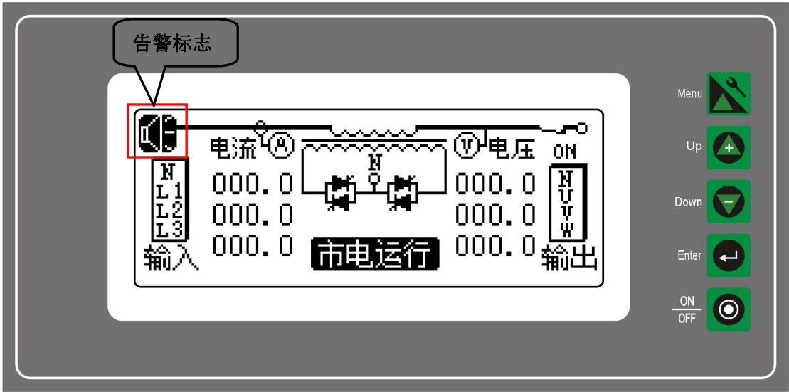
图 6.1 界面 1 (主界面)
