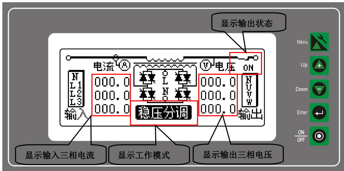
图 4 界面 1 (主界面)
