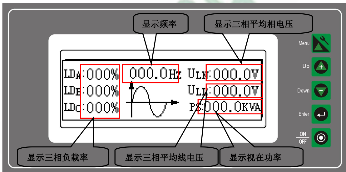
图 5 界面 2
